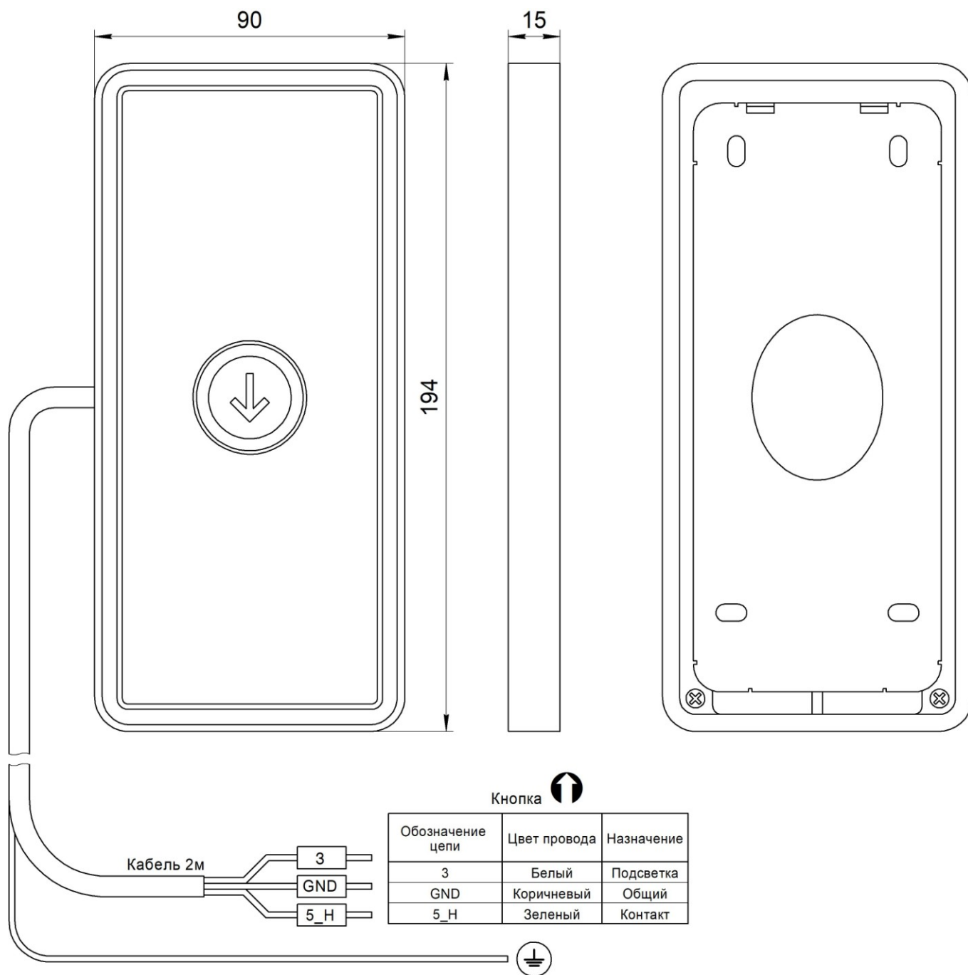
Рис.1 Внешний вид и габаритные размеры Вызывного поста ОБСИДИАН НШЕК.468381.217
